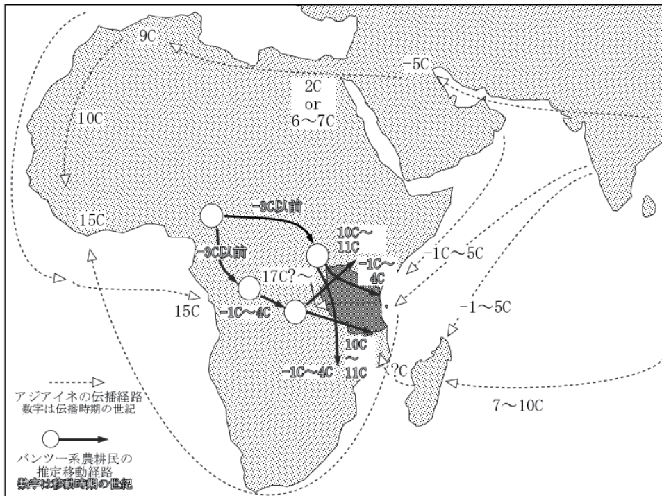
図1 アジアイネのアフリカ大陸への伝播ルートとバンツール系農耕民の移動経路 出所：Harlan (1992)、星川 (1996)、福田 (1997)、市川 (1997)、渡辺 (2009) の情報をもとに筆者作成
